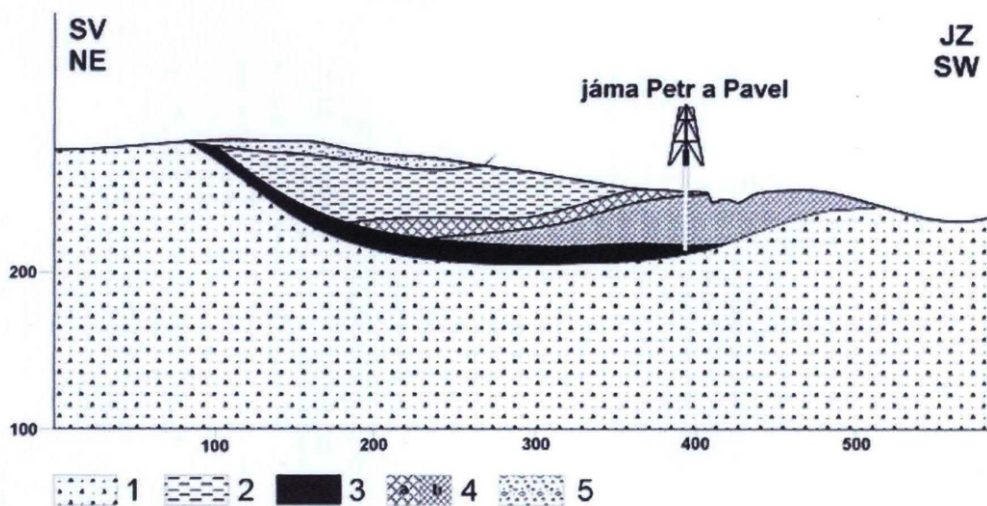
Obr. 4: Geologický řez C nechvalickou pánvičkou (Macůrek, Zelenka 1985)
