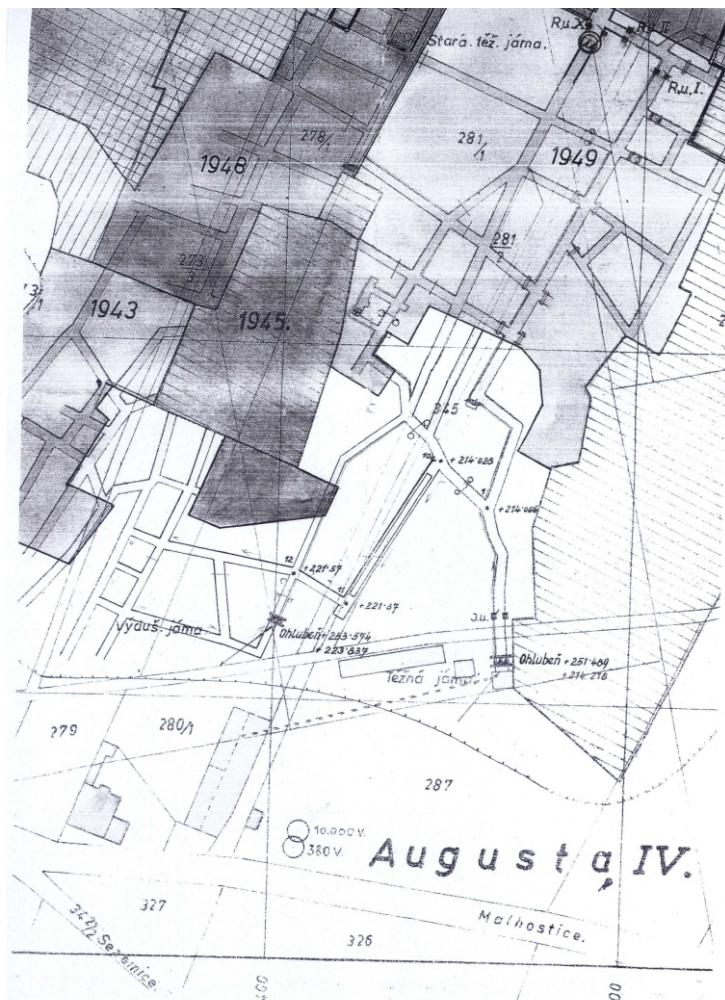
Mapa důlního díla Petr a Pavel - Nechvalice
